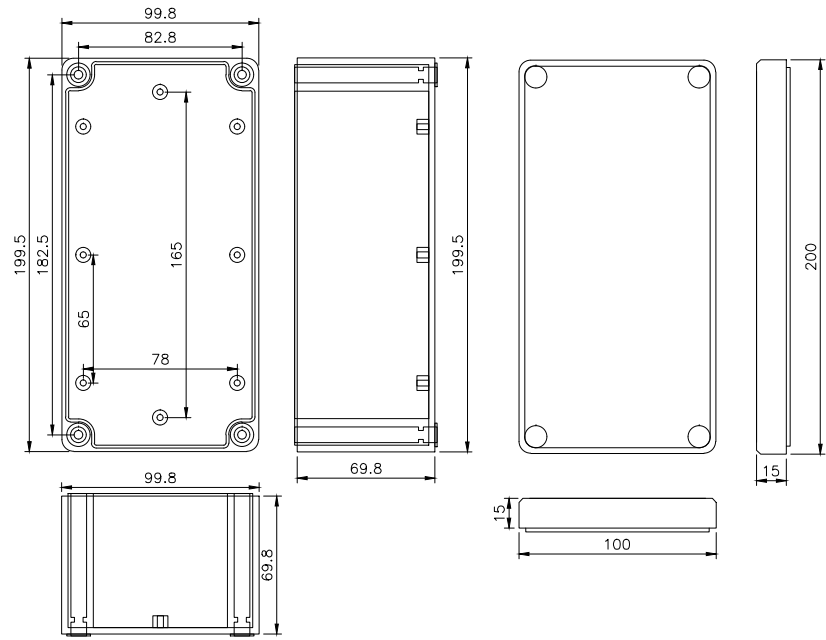
FINEBOX AB-1020-85
